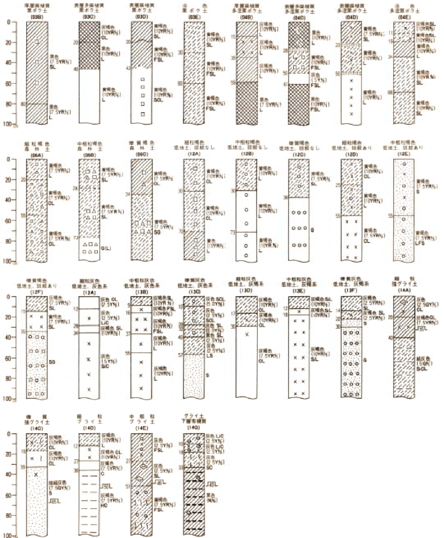
図 - 1 各土壌統群の代表土壌断面柱状図
